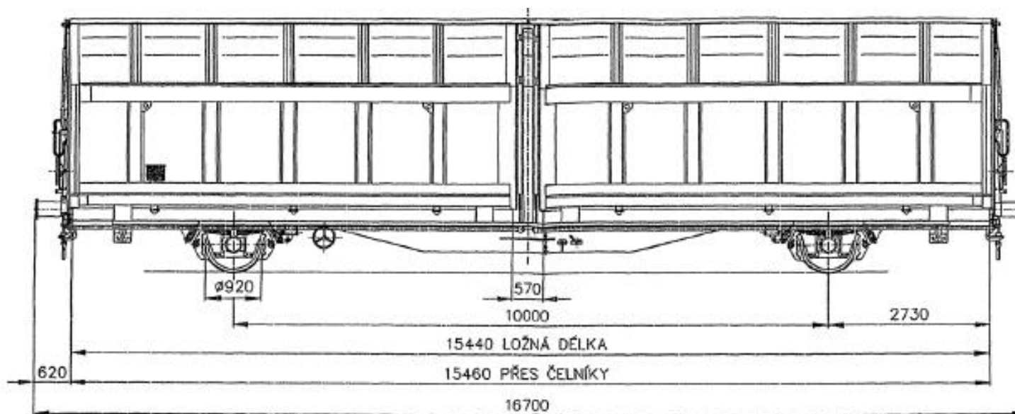
SVĚTLÝ PRŮŘEZ VOZU
